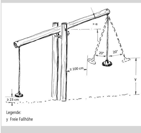
Abbildung 27 Einachsige Überkopf-Wippe (Typ 6)
