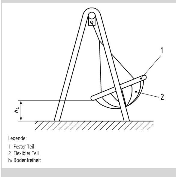
Abbildung 17 Bodenfreiheit bei Gruppenschaukelsitzen mit flexiblem Teil
