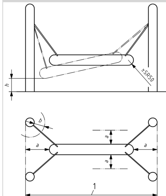
Abbildung 14 Beispiel eines schweren, abgehängten Balkens
