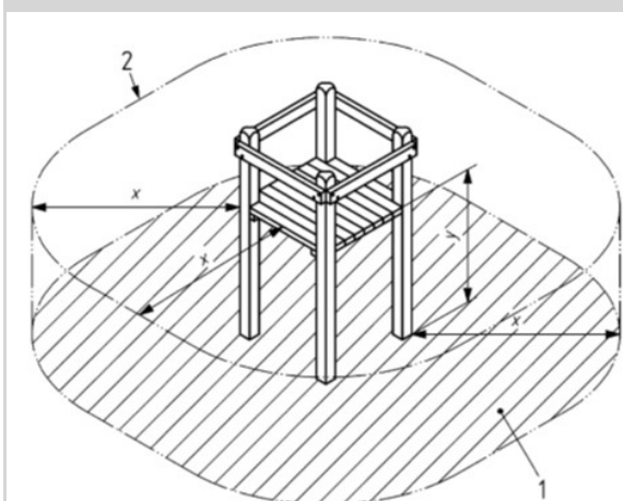
Abbildung 11 Beispiel Fallraum und Aufprallfläche einer Plattform
