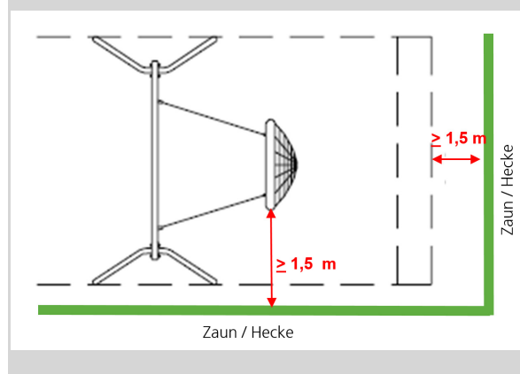
Abbildung 18 Empfehlung für das Aufstellen von Zäunen in der Nähe von Schaukeln
